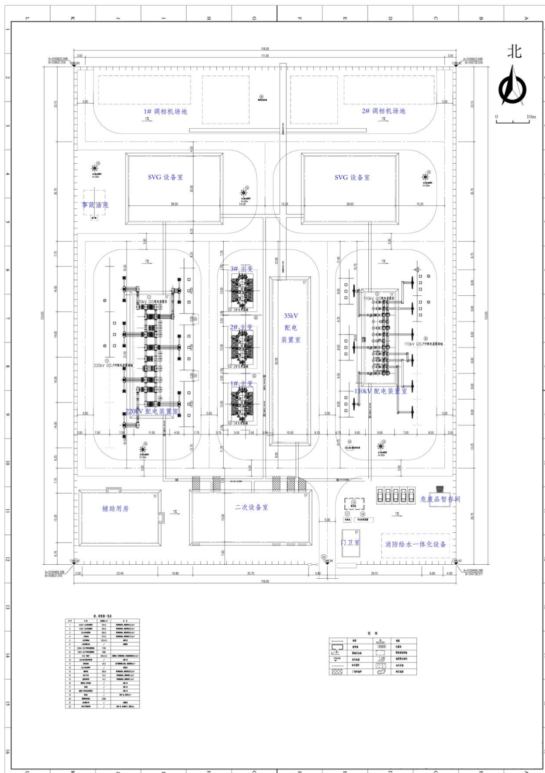
图 4-2 总平面布置图
